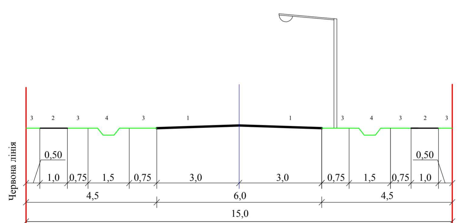
Вулиця Лісна Розріз 1-1
