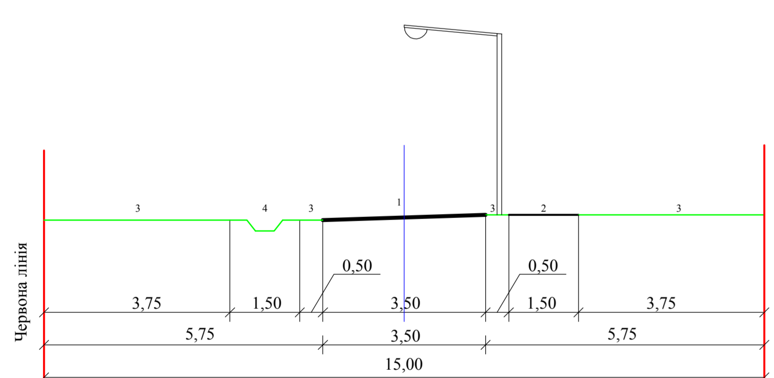
Житлова вулиця (Проїзд) Розріз 3-3
