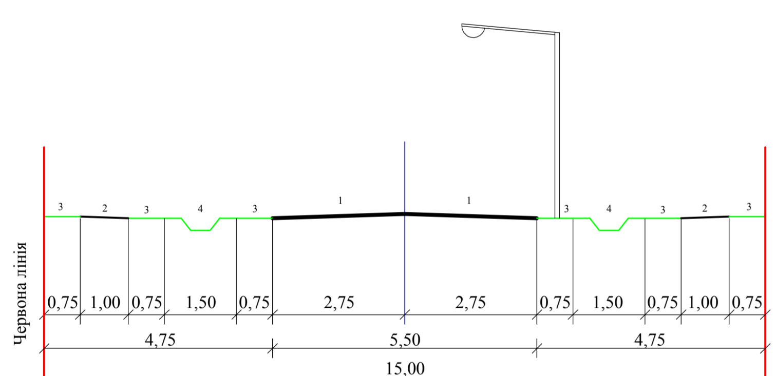
Вулиця Набережна Розріз 2-2
